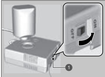
1 Schakelaar luchtcompressor
