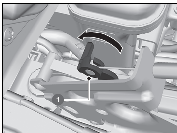
1 Ontgrendelingshendel
