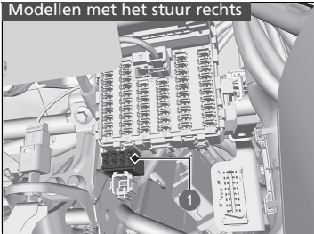
1 Zekeringkast B
